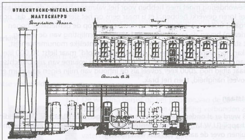
Utrechtse Waterleiding Maatschappij Ontwerp van het Baarnse pompstation. Bouwtekening uit ongeveer 1885.
