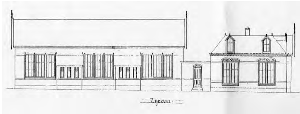
Een zijgevel op de bouwtekening van de R.K. Sint Aloysiusschool
