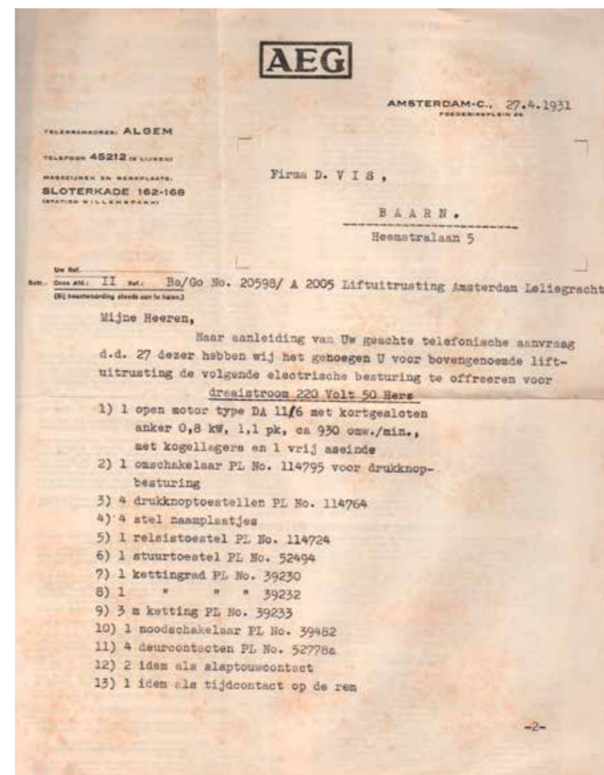
Afb. 3. Eerste pagina van een offerte van AEG uit 1931 voor de elektrische besturing voor draaistroom 220 Volt 50 Herz van een lift. (Archief Liftenfabriek Baarn)
